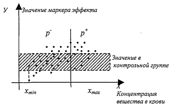
Рис. 2. Схема представления выборочных данных из двух частей
